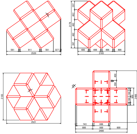
名 称 六脚ブロックA0.80形 体 積 3.516m 3 参考質量 8.087t 型枠面積 15.41m 2
