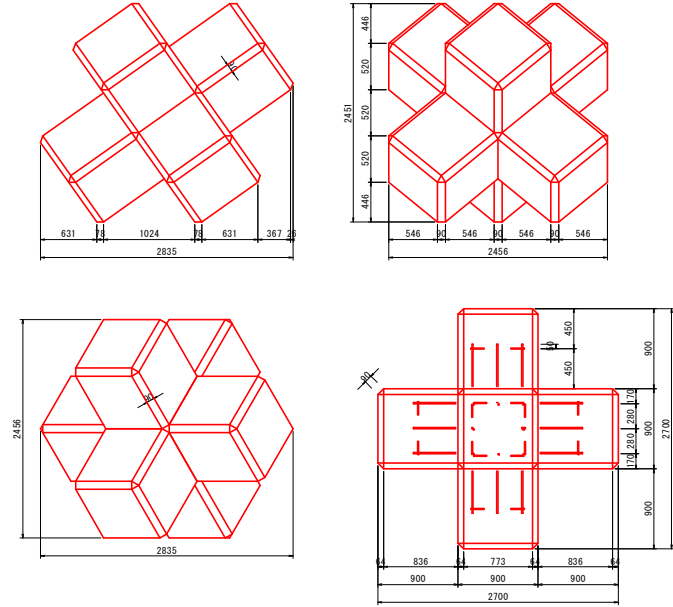
名 称 六脚ブロックA0.90形 体 積 5.006m 3 参考質量 11.514t 型枠面積 19.50m 2
